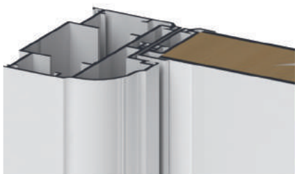
detalle del núcleo macizo en contrachapado
